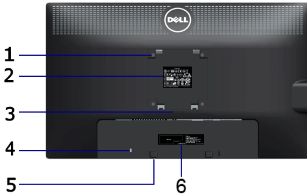
後方図
